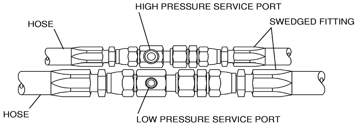
VIEW A-A
